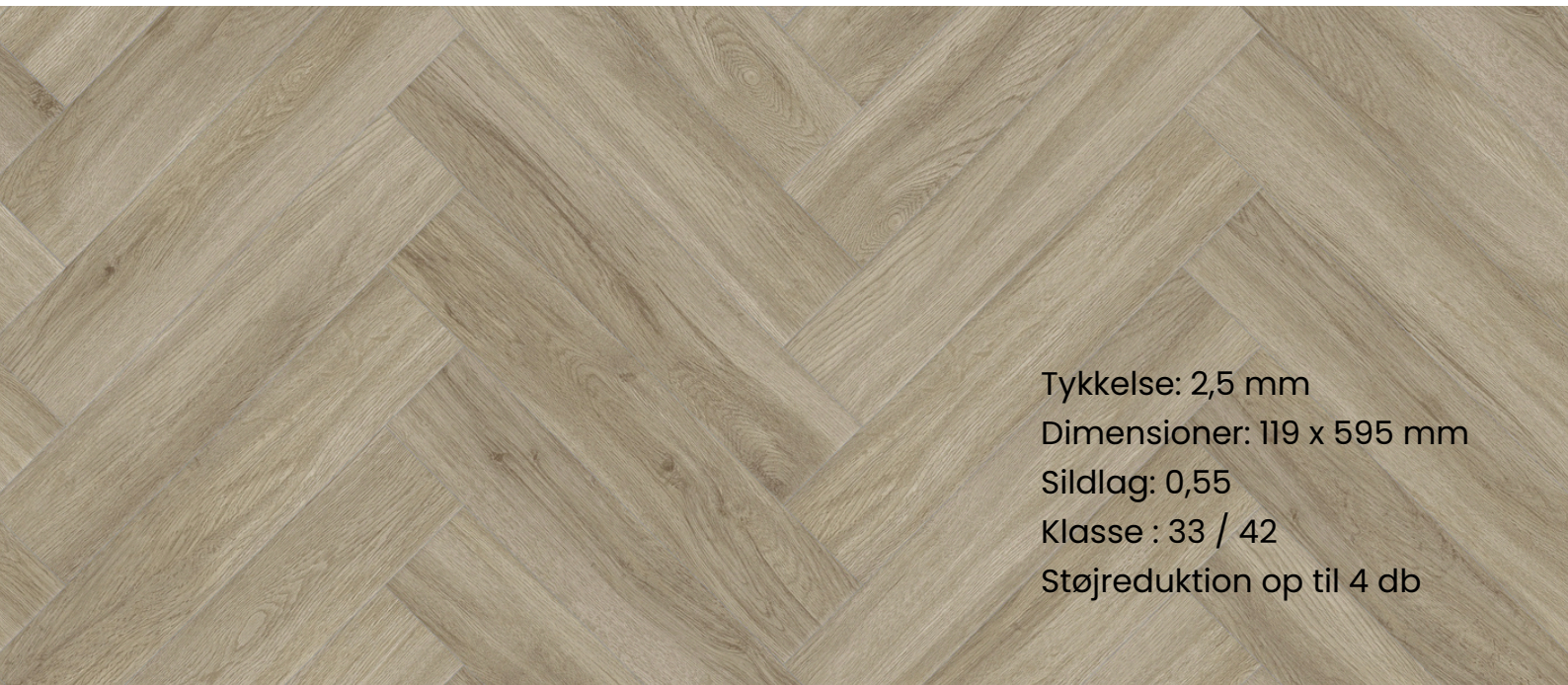
LVT DRYBACK GRÅ SILDEBEN 8850 ( 918850 )
