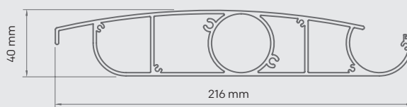
Tværsnit af lamel
